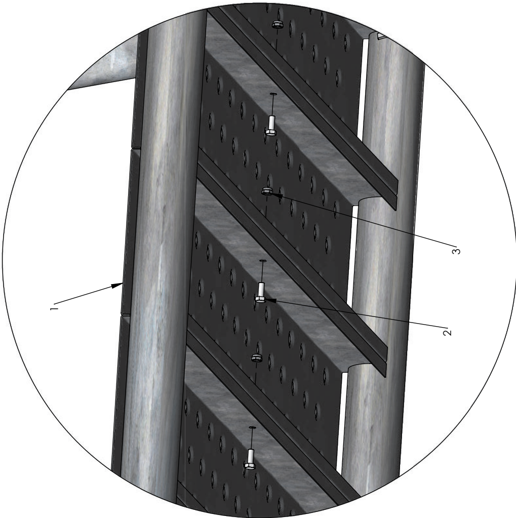
DÉTAIL C ECHELLE 1 : 4
