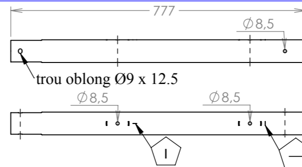
N° Pièce : MIRADOR2400T16 Matière : SENDZIMIR Epaisseur : 1.5 mm Quantité : 2 Poids : 1.67 Kg
