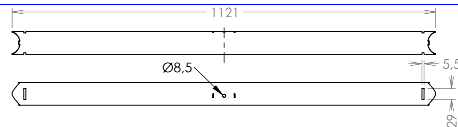
N° Pièce : MIRADOR2400T19 Matière : SENDZIMIR Epaisseur : 1.5 mm Quantité : 2 Poids : 2.38 Kg
