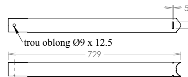
N° Pièce : MIRADOR2400T17 Matière : SENDZIMIR Epaisseur : 1.5 mm Quantité : 1 Poids : 1.54 Kg
