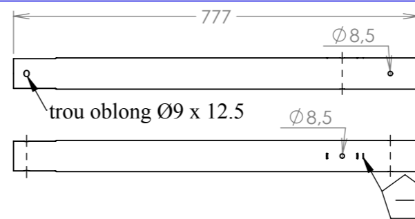
N° Pièce : MIRADOR2400T15 Matière : SENDZIMIR Epaisseur : 1.5 mm Quantité : 2 Poids : 1.67 Kg
