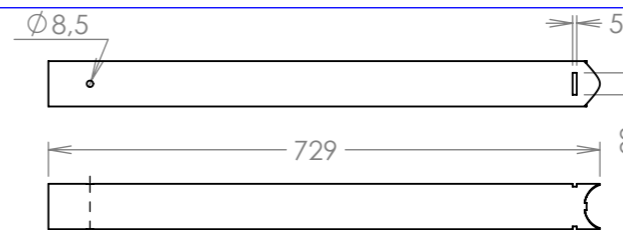
N° Pièce : MIRADOR2400T18 Matière : SENDZIMIR Epaisseur : 1.5 mm Quantité : 1 Poids : 1.55 Kg
