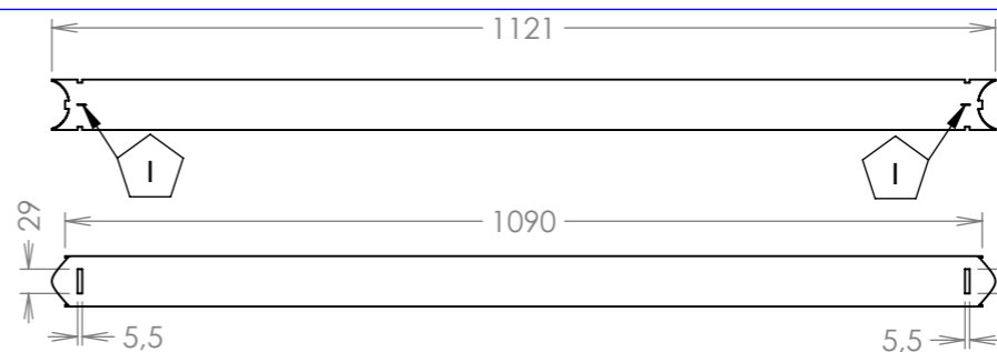
N° Pièce : MIRADORT08 Matière : SENDZIMIR Epaisseur : 1.5 mm Quantité : 1 Poids : 2.38 Kg
